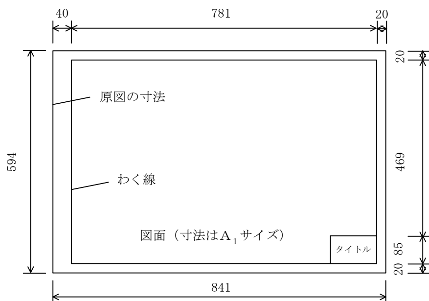
図－１ 図面寸法（単位 mm）
