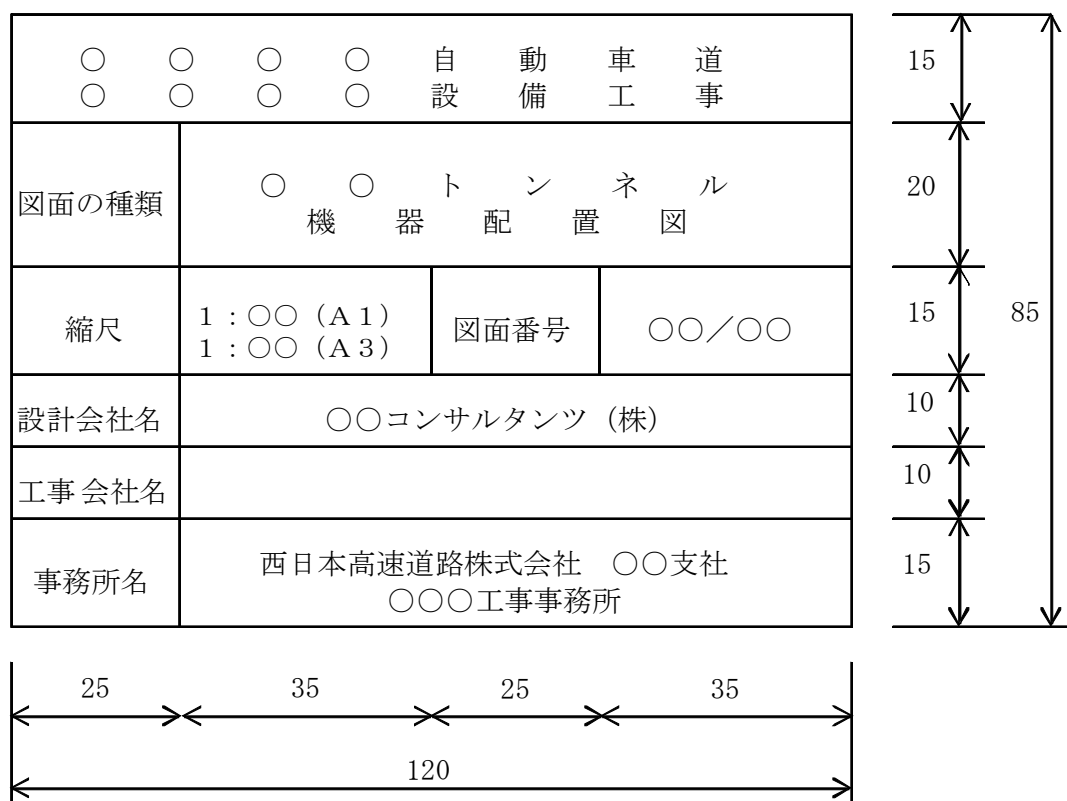
図－２ 図面タイトル寸法（単位 mm）
